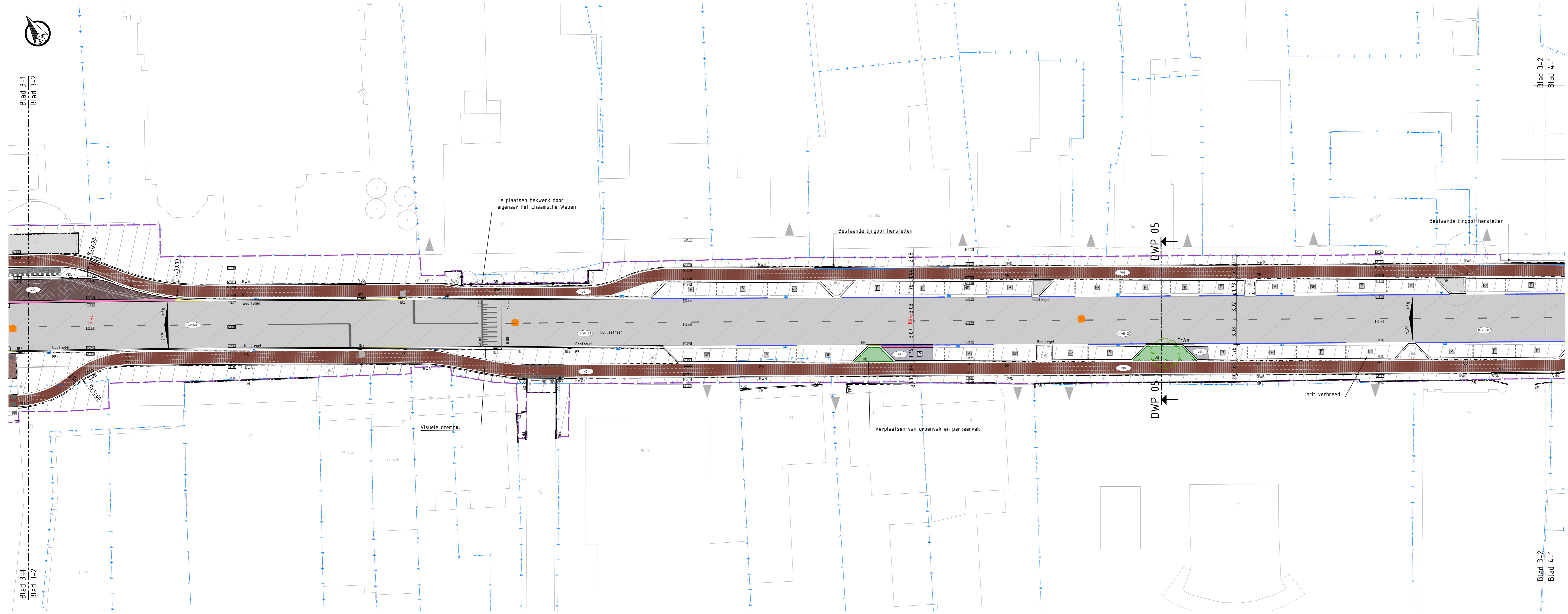
SITUATIE: BLAD 3-2 SCHAAL 1:200
