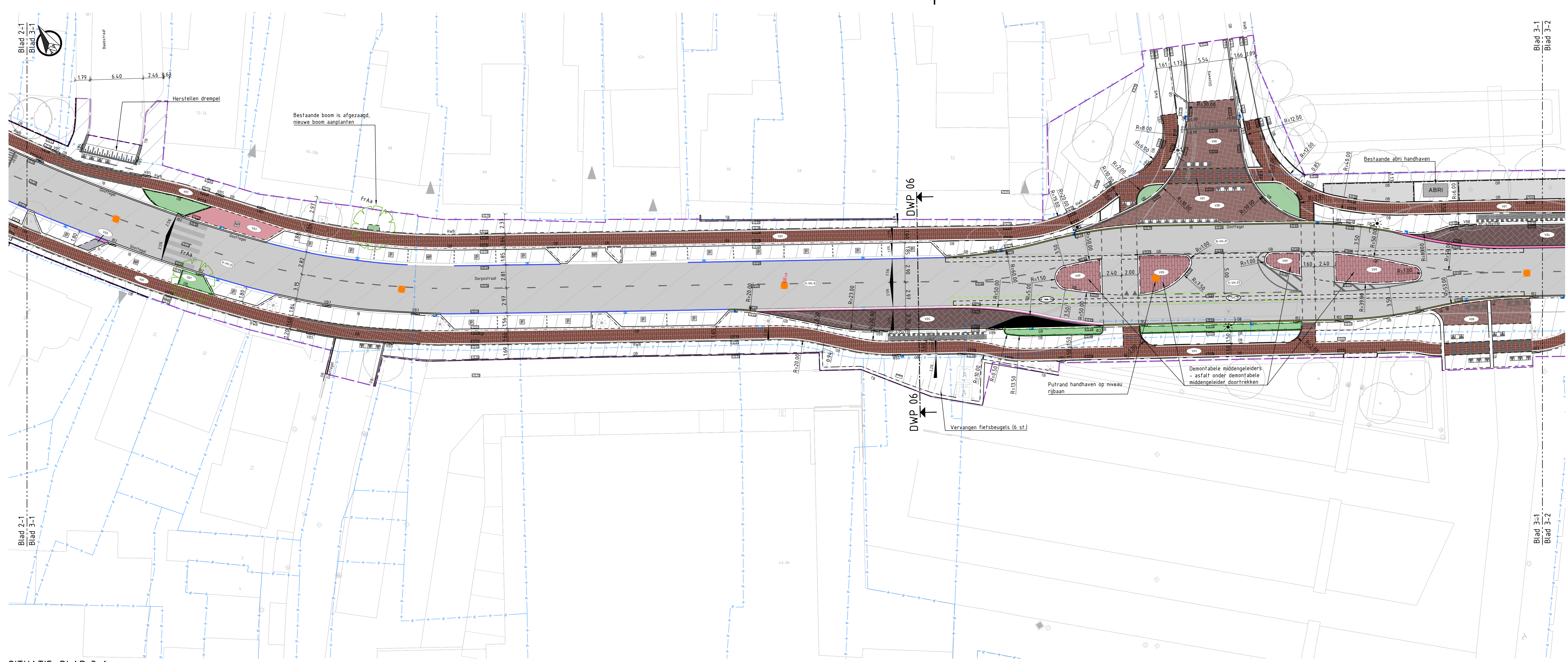
SITUATIE: BLAD 3-1 SCHAAL 1:200
