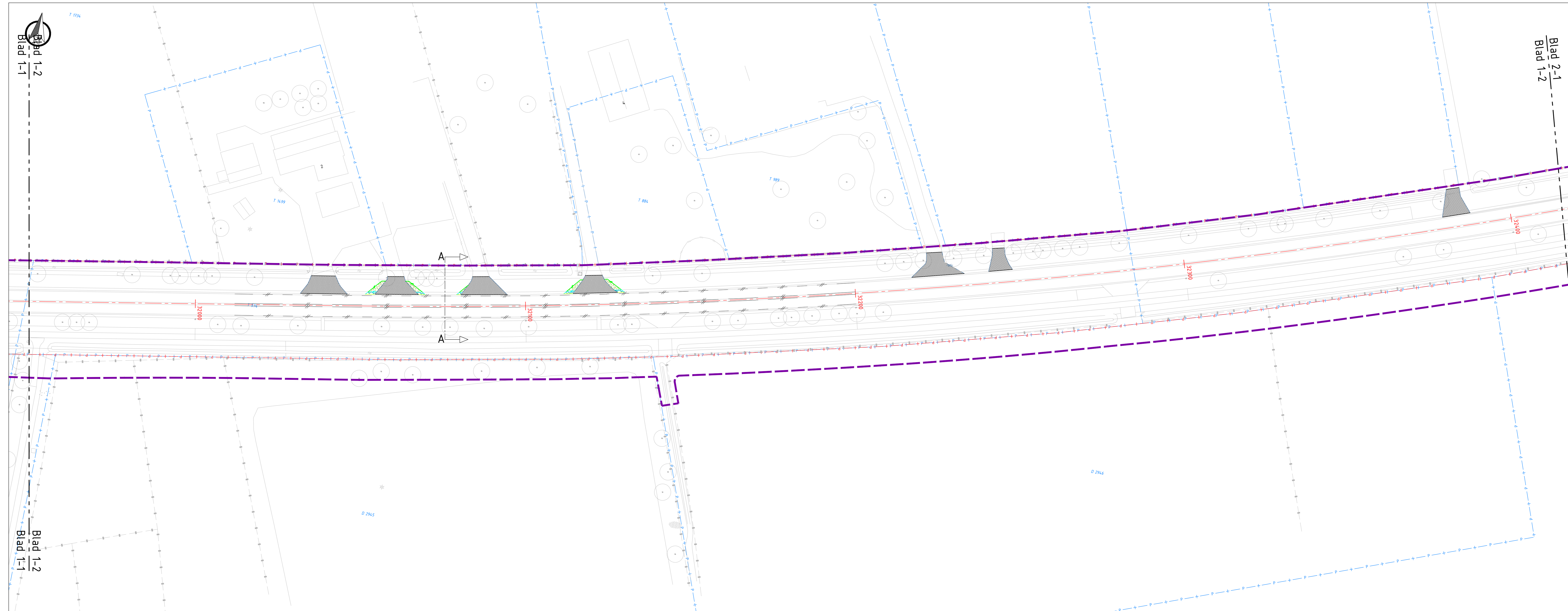
SITUATIE: BLAD 1-2 SCHAAAL 1:500
