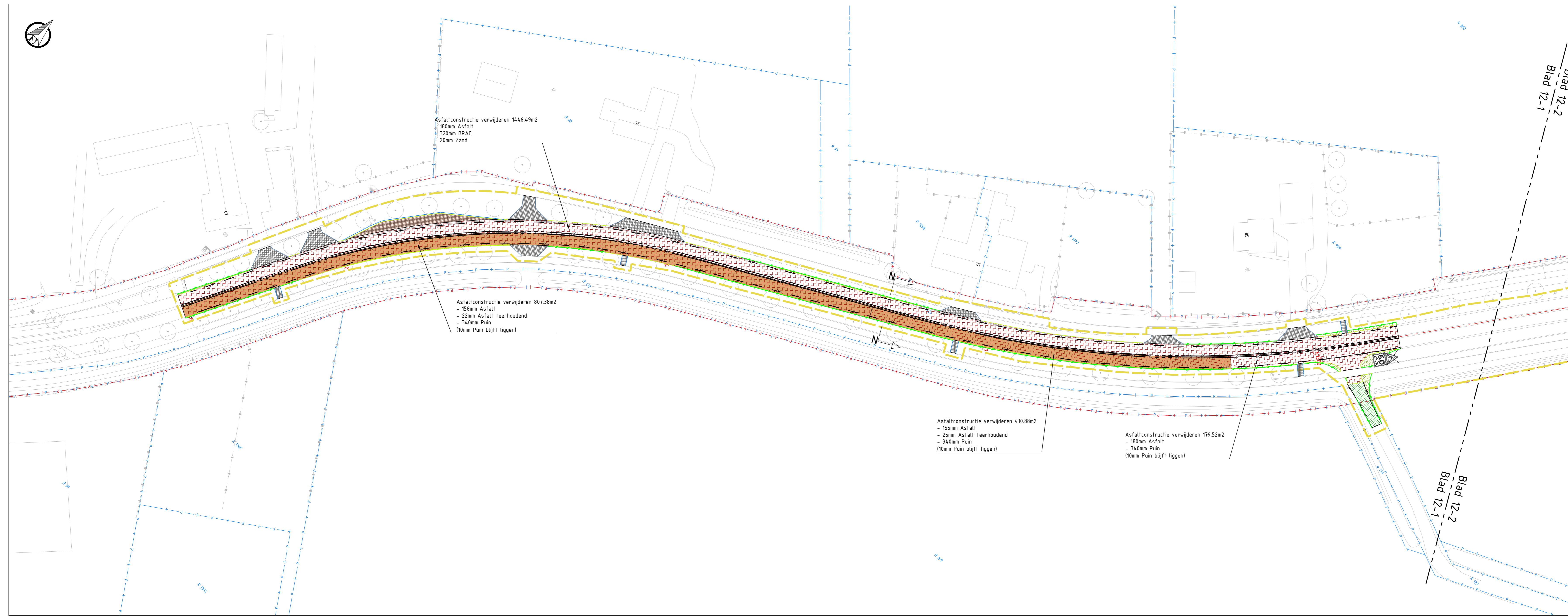
SITUATIE: BLAD 12-1 SCHAAAL 1:500
