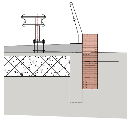
Aanzicht kopzijde brugdekrand
