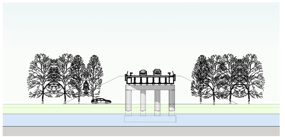
Dwarsdoorsnede tussensteunpunt
