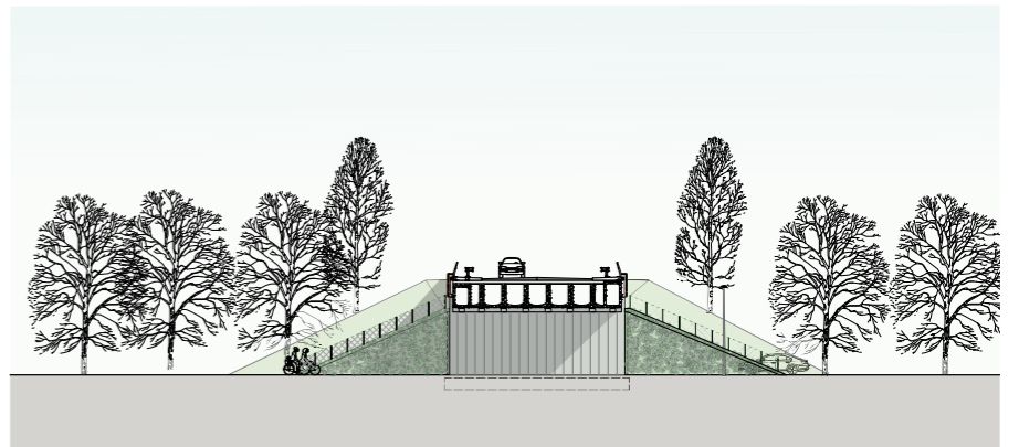
Dwarsdoorsnede aanzicht landhoofd Koekoekse dijk
