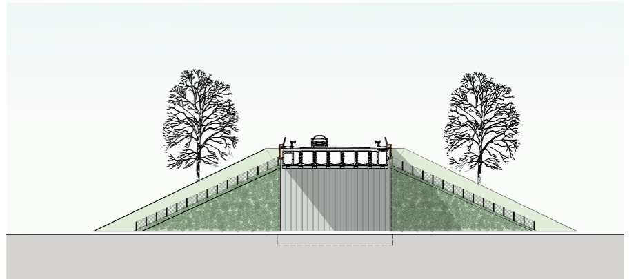
Dwarsdoorsnede, aanzicht landhoofd Schansdijk
