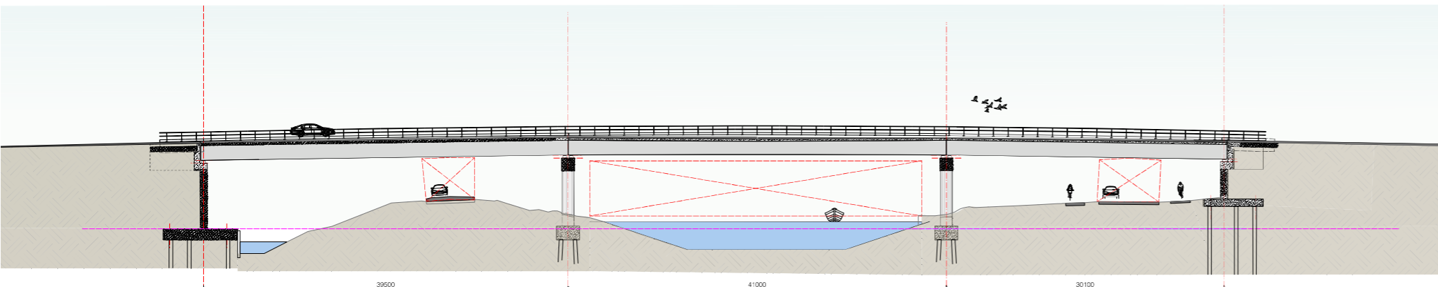
Langsdoorsnede
